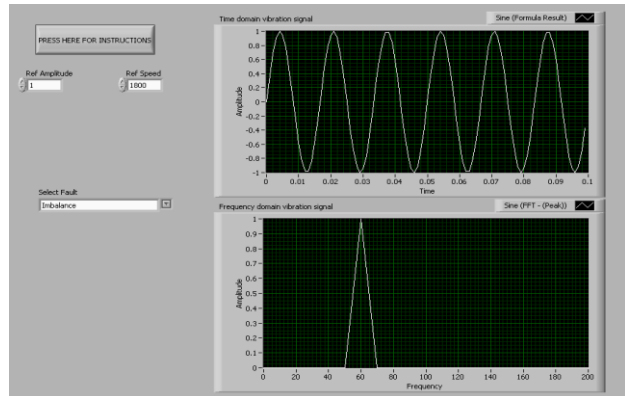
Fig. 6 Pure Imbalance
